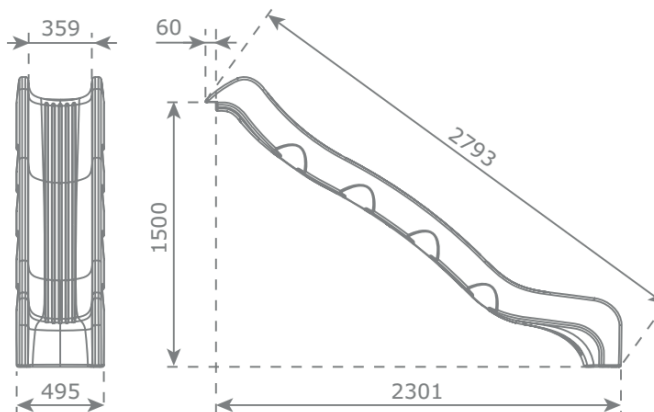
Altura de plataforma 1500 mm
